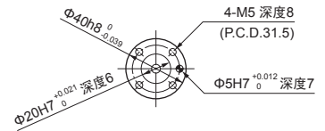
底座安装面（从上面观察）
