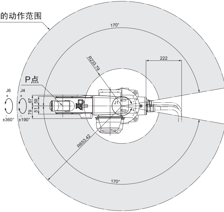
工具安装面详图（箭头视图A）
