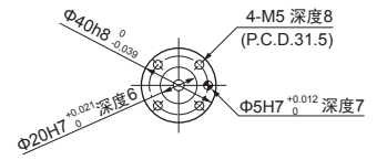
底座安装面（从上面观察）
