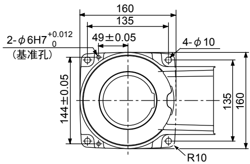
底座安装尺寸 (俯视)
