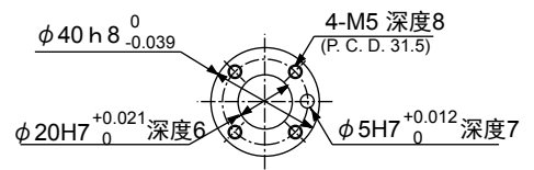
工具安装面详图 (箭头视图A)
