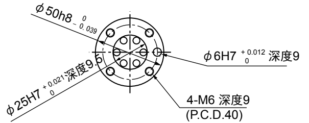
工具安装面详图 (A视图)
