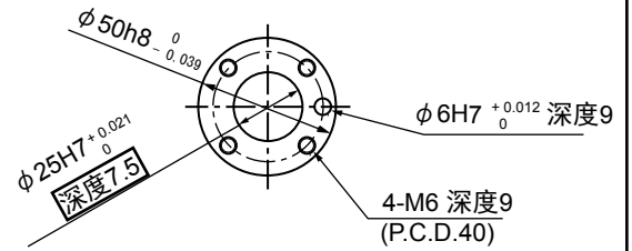
工具安装面详图 (A视图)
