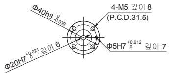
틀 장착면 상세 (A에서 봤을 때)
