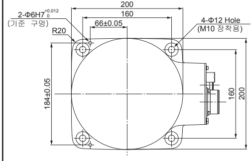
베이스 장착면 (상면에서)
