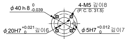
틀 장착면 상세 (화살표A)
