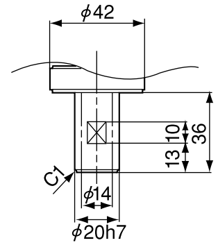
ツール取付面詳細(矢視 D)
