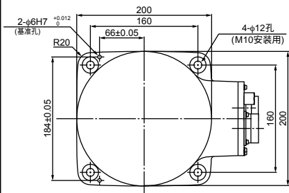
底座安装面 (从上面看)
