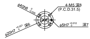
底座安装面 (从上面看)
