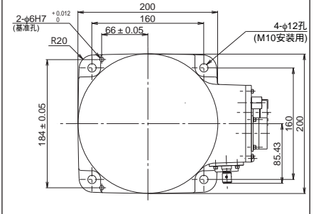
底座安装面 (从上面看)
