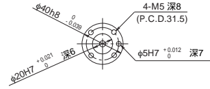
底座安装面 (从上面看)
