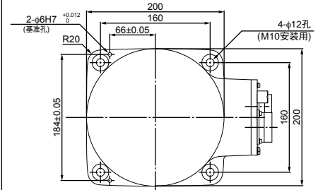
底座安装面 (从上面看)
