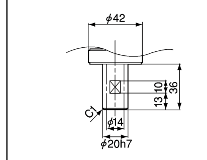
ツール取付面詳細 (矢視D)
