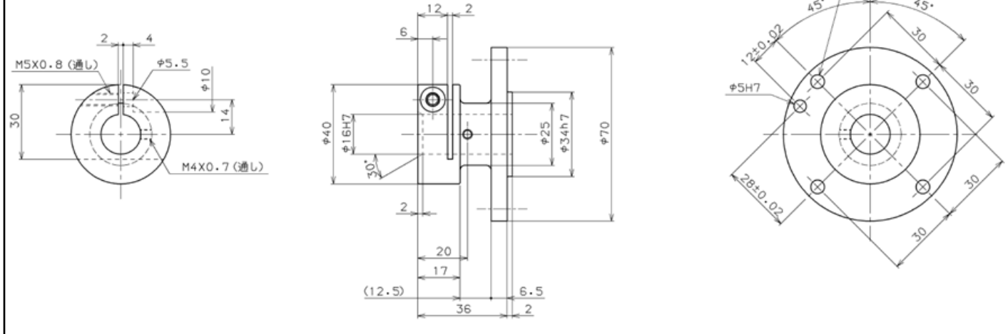
法兰（选件）安装图纸
