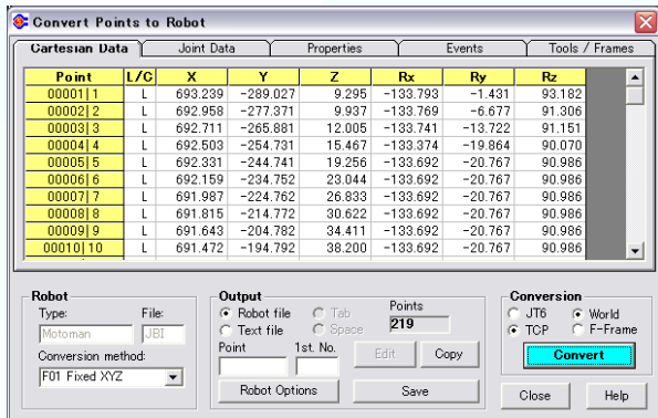
コンパートフォーム、ロボットファイル出力(各軸変位、パスポイント座標、等)
