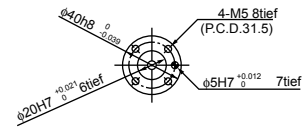
Detailzeichnung der Grundmontageseite (Ansicht von oben)
