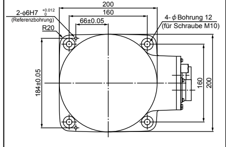
Detailzeichnung der Grundmontageseite (Ansicht von oben)
