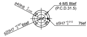
Detailzeichnung der Grundmontageseite (Ansicht von oben)
