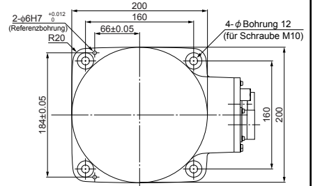
Detailzeichnung der Grundmontageseite (Ansicht von oben)
